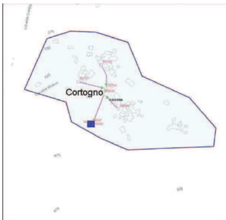
SCHEMA RETICOLO FOGNARIO
