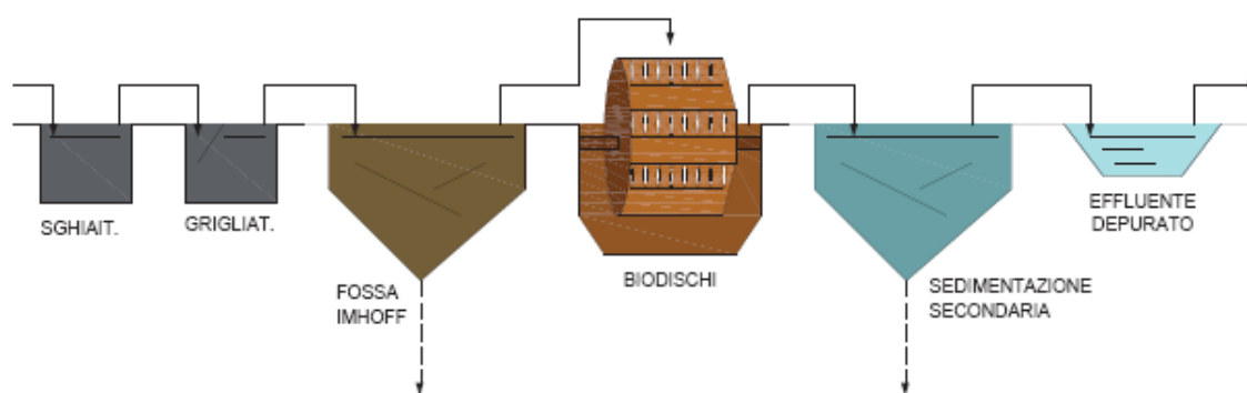
SCHEMA IMPIANTO
