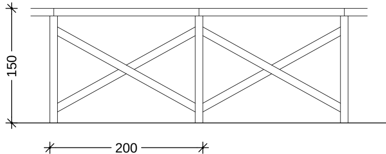
PARTICOLARE STACCIONATA IN LEGNO STATO DI PROGETTO Scala 1:50
