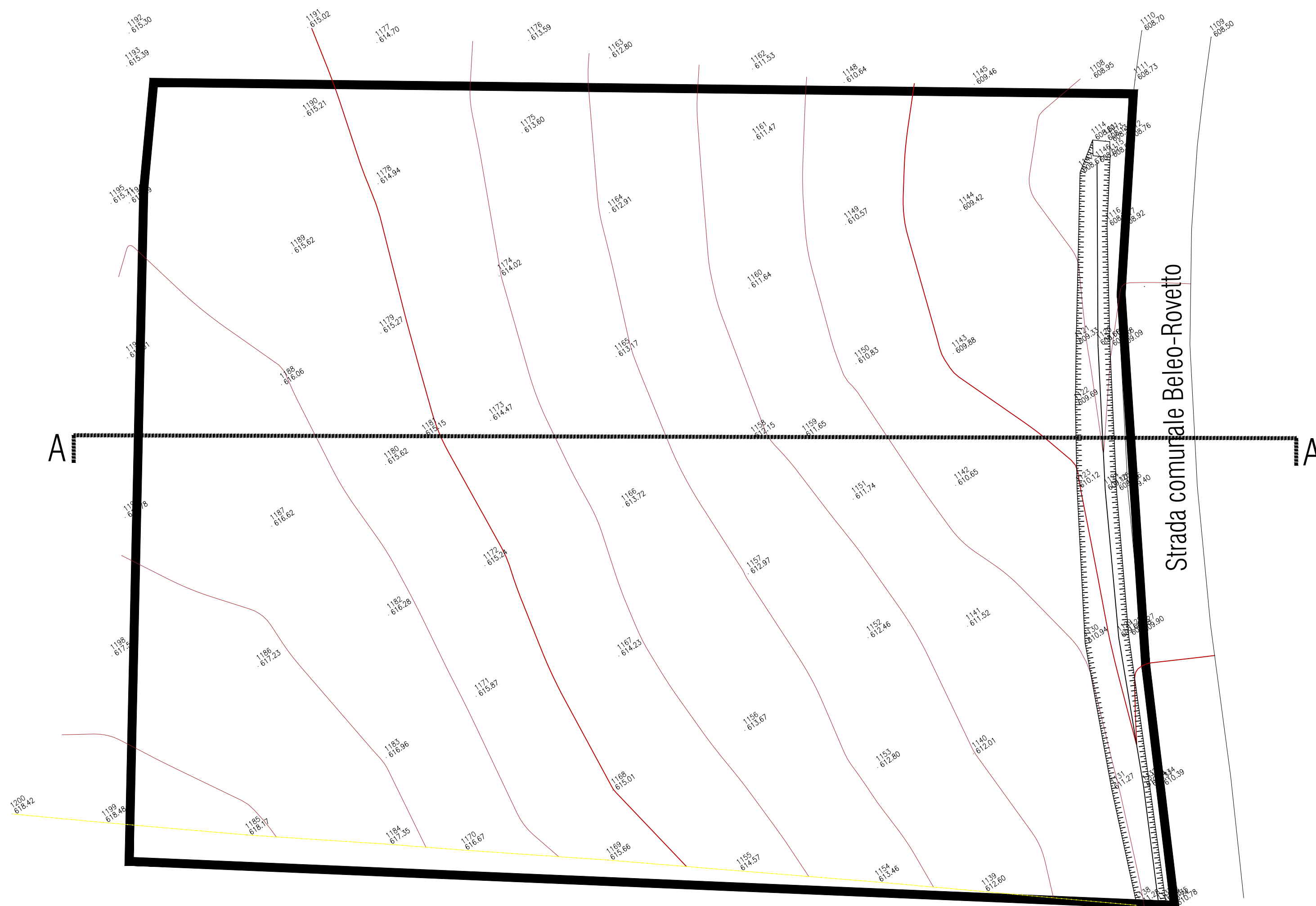
PLANIMETRIA CON RILIEVO PLANI-ALTIMETRICO DELLO STATO DI FATTO Scala 1:200
