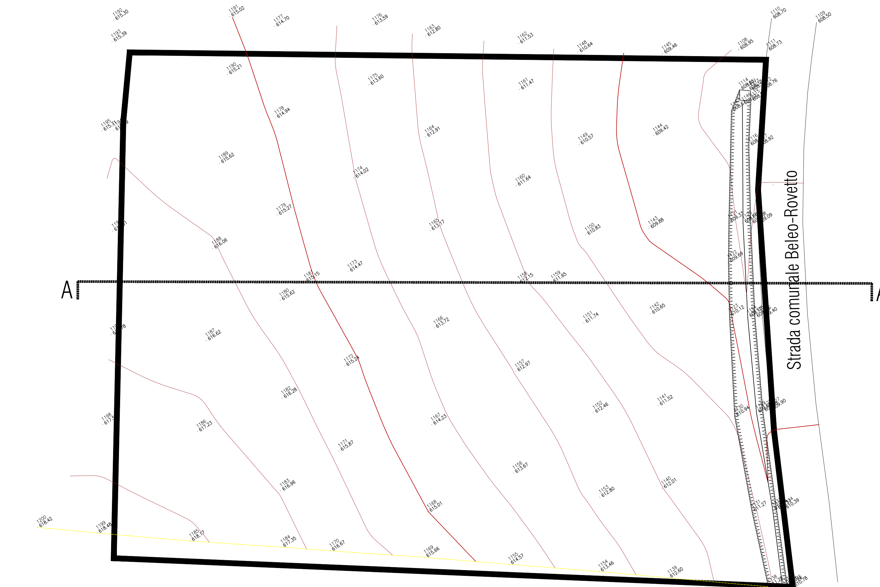
PLANIMETRIA CON RILIEVO PLANI-ALTIMETRICO DELLO STATO DI FATTO Scala 1:200
