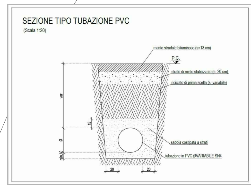
Particolare costruttivo
